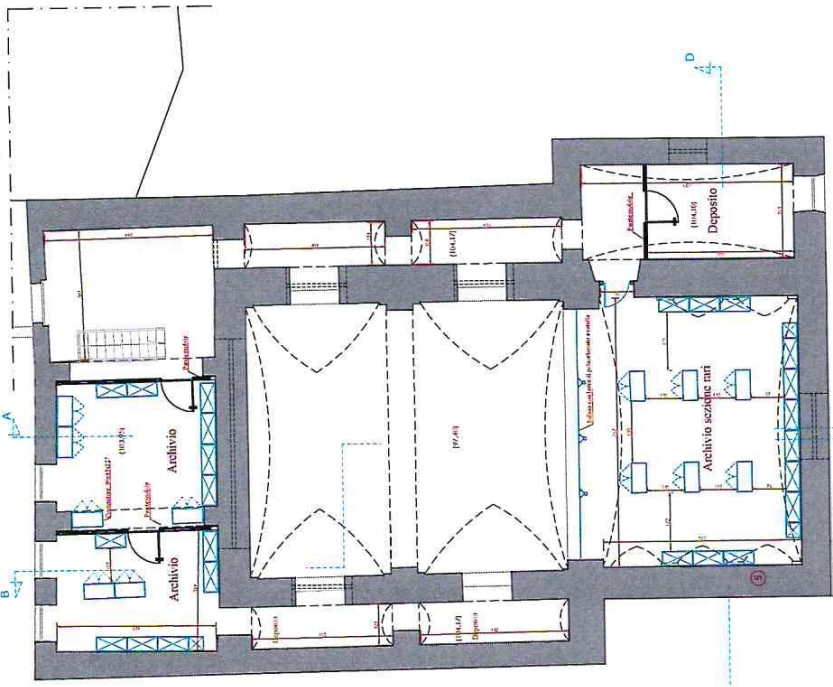
PIANTA PIANO PRIMO rapp. 1:50
