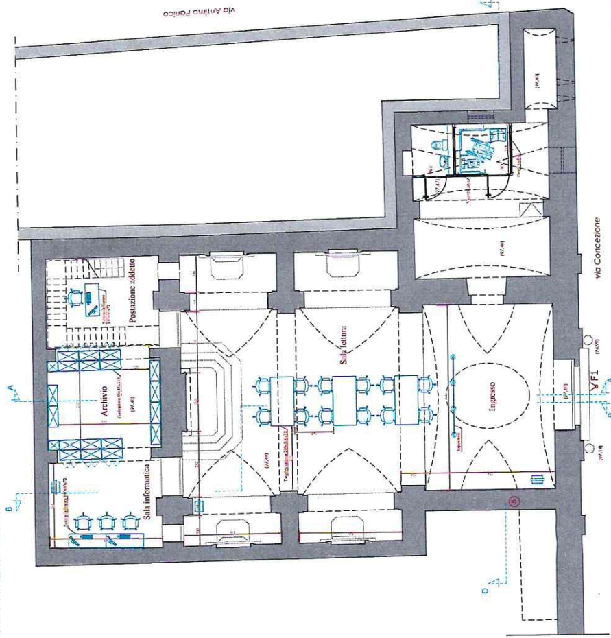
PIANTA PIANO TERRA rapp. 1:50
